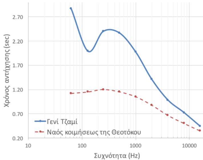
Σχήμα 1. Χρόνος αντήχησης χώρων λατρείας που μελετήθηκαν στα πλαίσια του παρόντος έργου συναρτήσει της συχνότητας.
