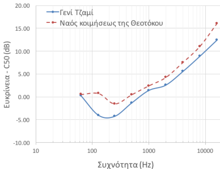
Σχήμα 2. Ακουστική ευκρίνεια (C50) χώρων λατρείας που μελετήθηκαν στα πλαίσια του παρόντος έργου συναρτήσει της συχνότητας.
