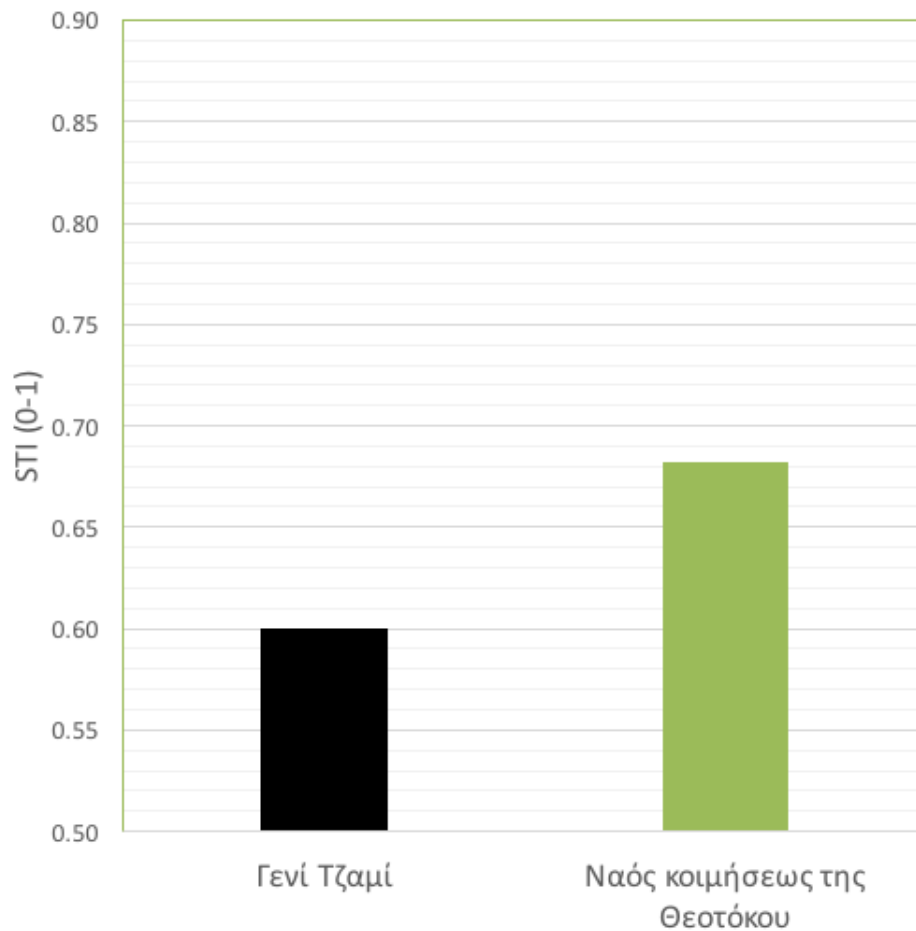
Σχήμα 3. STI χώρων λατρείας που μελετήθηκαν στα πλαίσια του παρόντος έργου.
